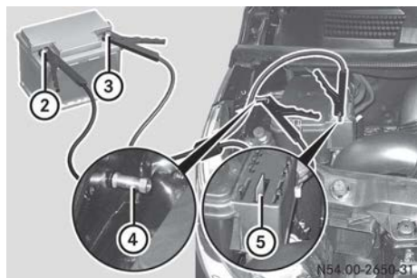
Schéma de connexion
